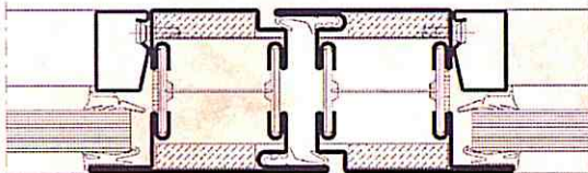
Janisol 2 EI30 (F30/T30)
