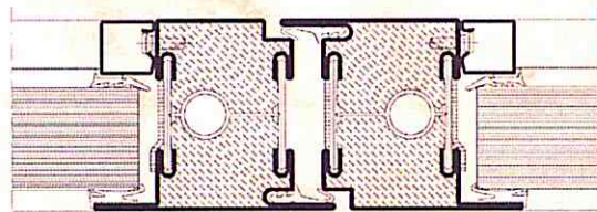
Janisol 4 EI90 (F90/T90)
